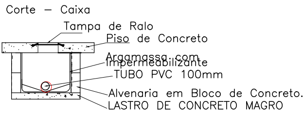
Corte - Caixa
