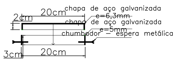
Corte - Tampa
