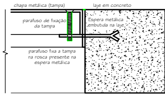
Detalhe Fixação
