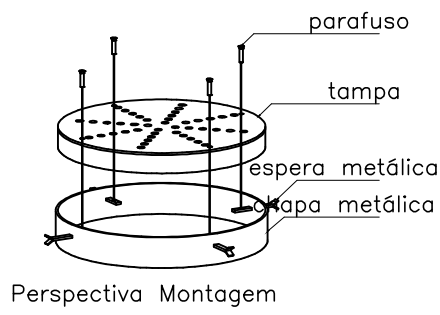
Perspectiva Montagem
